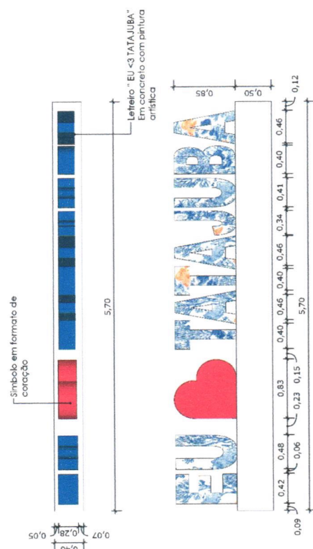
DETALHE LETREIRO 1:25
